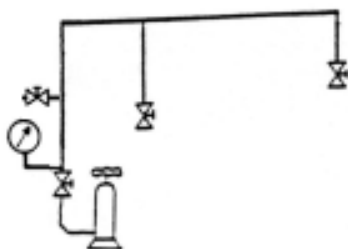
Εικόνα 10.2 Δοκιμή στεγανότητας
