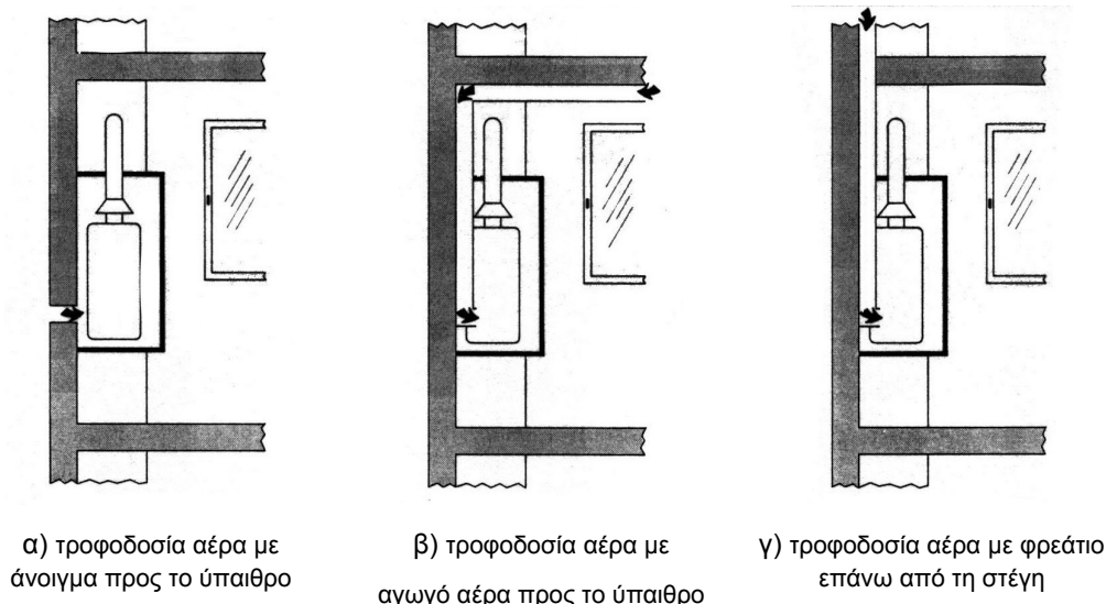
Εικόνα 8.5 Παραδείγματα για την εγκατάσταση συσκευών του τύπου B 1 ή B 4 σε ιδιαίτερο περίβλημα
