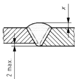
Εικόνα 1.1 Πρότυπη κατατομή ραφής για σωλήνες και εξαρτήματα ραφών
