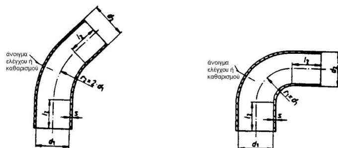
Εικ.9.4 Στοιχεία μορφής καπναγωγών από μέταλλο
