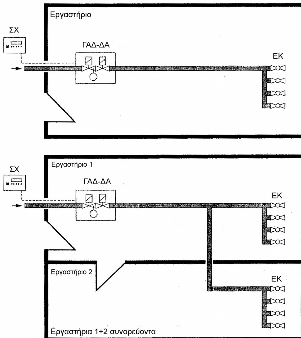
Εικόνα 2 Παράδειγμα δικτύου σωληνώσεων σε εργαστήριο και γειτονικούς χώρους εργαστηρίων
