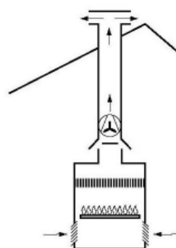
B 44 με ανεμιστήρα μετά την ασφάλεια ροής
