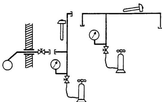
Εικόνα 10.1 Δοκιμή αντοχής
