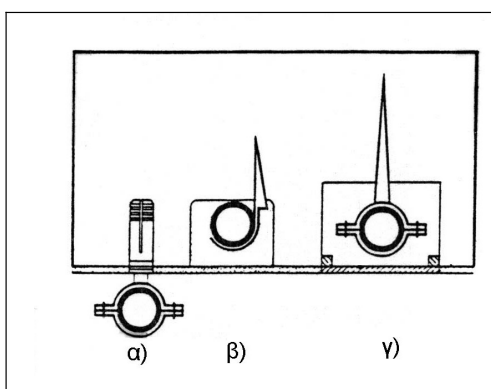
Εικόνα 1.9 Παραδείγματα εγκατάστασης των σωληνώσεων
