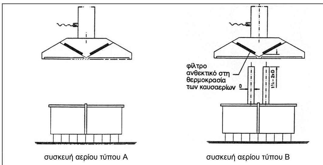
Εικόνα 13.1 Απαγωγή καυσαερίων συσκευών αερίου τύπου Α μέσω χοανών εξαερισμού
