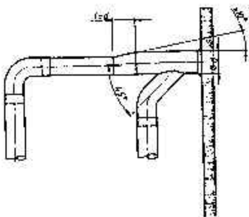
Εικόνα 11.1 Σχεδιασμός κοινού καπναγωγού
