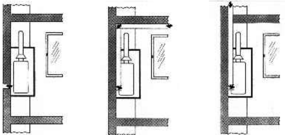
Εικόνα 10.5 Παραδείγματα για την εγκατάσταση συσκευών του τύπου B 1 ή B 4 σε ιδιαίτερο περίβλημα
