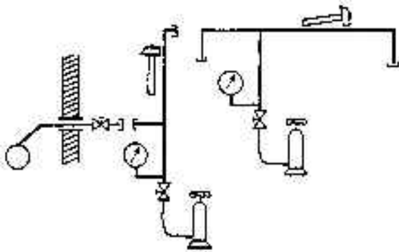
Εικόνα 12.1 Δοκιμή αντοχής
