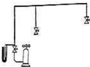
Εικόνα 12.2 Δοκιμή στεγανότητας
