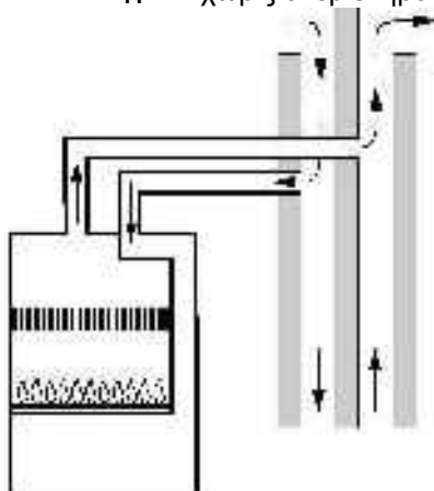
C41 χωρίς ανεμιστήρα
