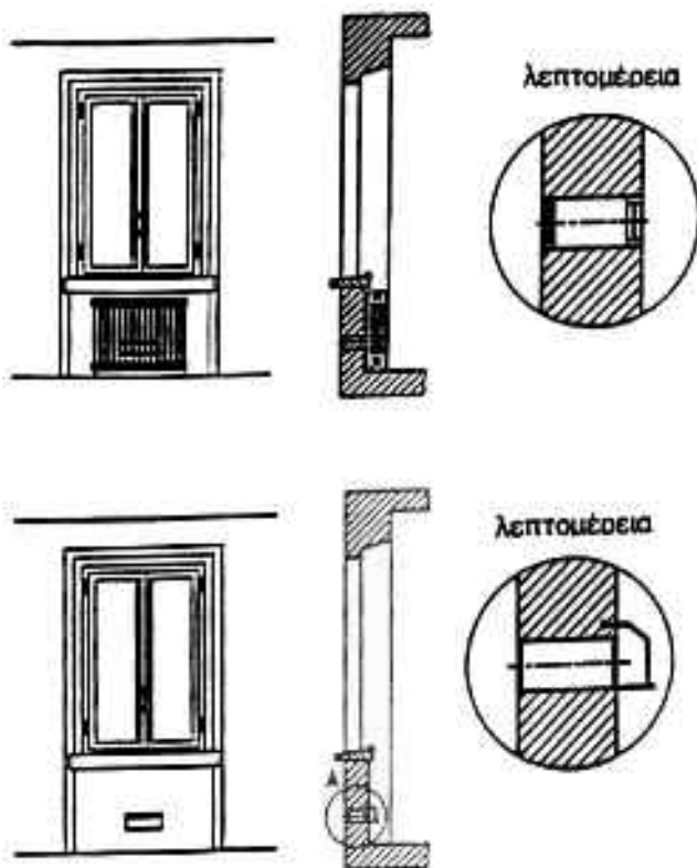
Εικόνα 10.3 Παραδείγματα θέσεων ανοιγμάτων τροφοδοσίας αέρα καύσης
