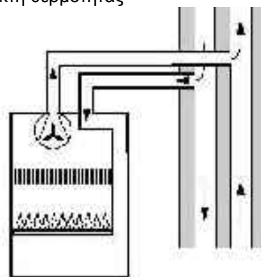
C42 με ανεμιστήρα μετά τον εναλλάκτη θερμότητας
