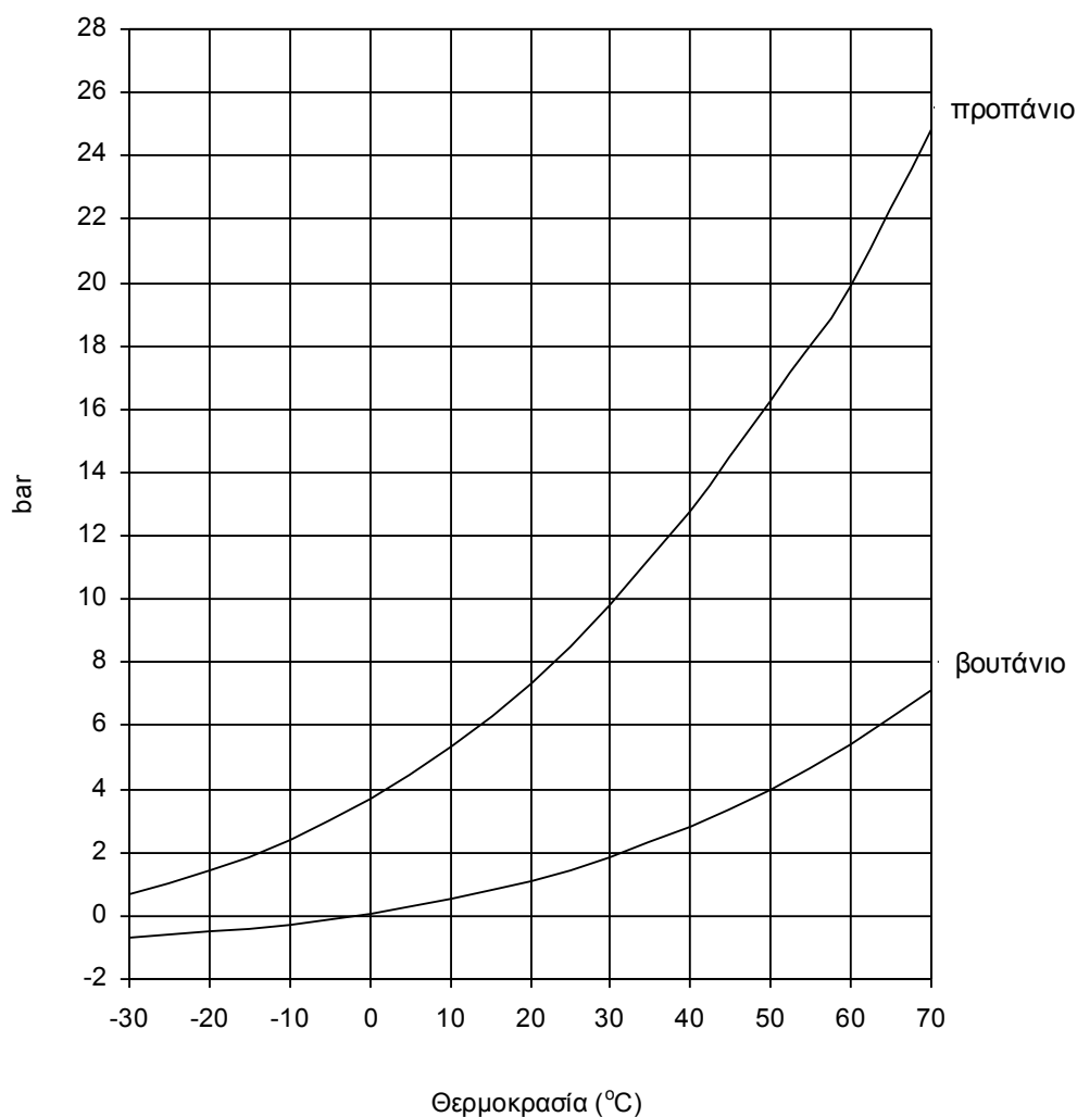
Εικ. 1 Καμπύλες (υπερ)πίεσης ατμών
