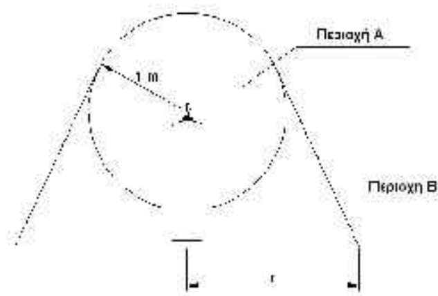
Εικόνα 6.1 Επικίνδυνες περιοχές φιαλών υγραερίου
